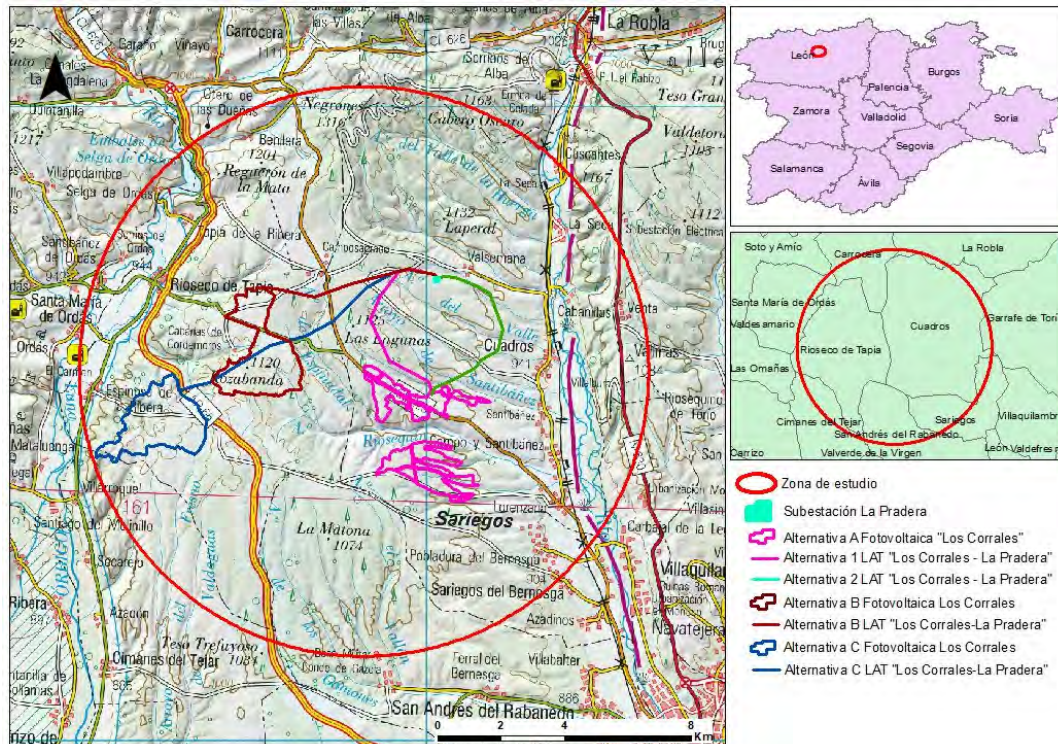
Figura 2.1. Alternativas de parcelas contempladas en la implantación de la planta solar fotovoltaica Los Corrales.
